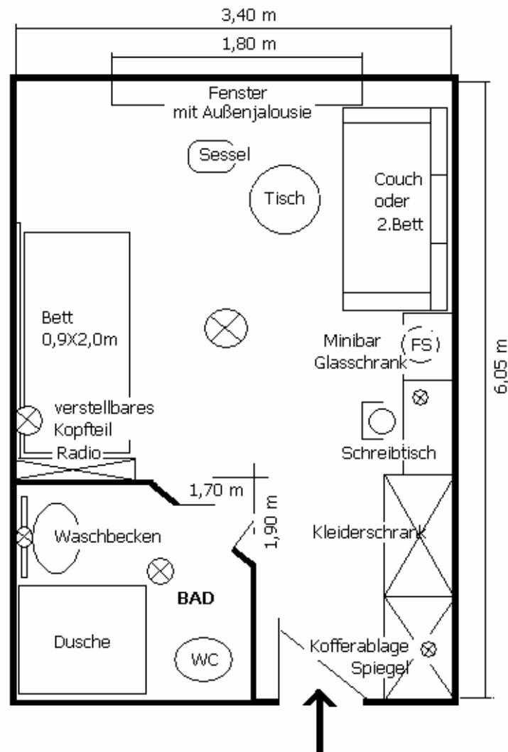
Einzelzimmer / Zweibettzimmer
